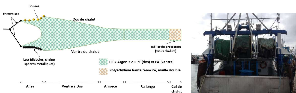
A gauche chalut de fond - Vue de profil (Source : IVAMER) ; à droite : Navire armé de chaluts (Source : IVAMER)
