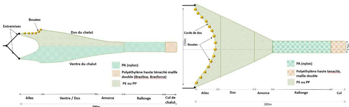
Chalut pélagique – à Gauche : Vue de profil ; à droite : vue du dessus (Source : IVAMER)
